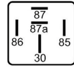
DNI8133 RELAY 5 TERMINALES 12V-40/20A SIN SOPORTE ACCESORIOS /VENTILADOR RADIADOR (MEGANE, CLIO, SCENIC, CITROEN) BOBINA CON DIODO) PARA:RENAULT SCENIC, CLIO, MEGANE
