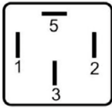
DNI8132 RELAY AUXILIAR 4 TERMINALES SIN SOPORTE 12V 60A PARA: CLIO SCENIC, MEGANE
