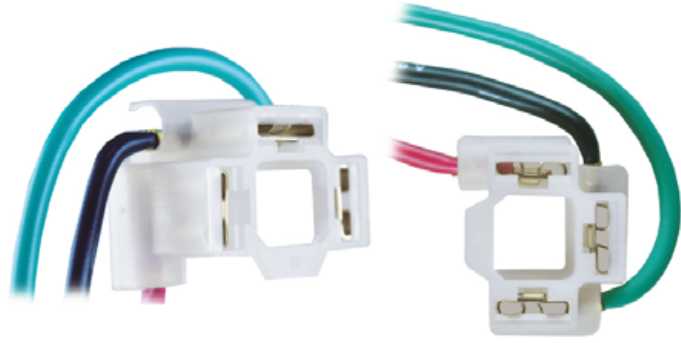
SU1 SOCKET DE UNIDAD CURVO CABLE CENTELSA No. 16 EMPAQUE: 20 UND.
