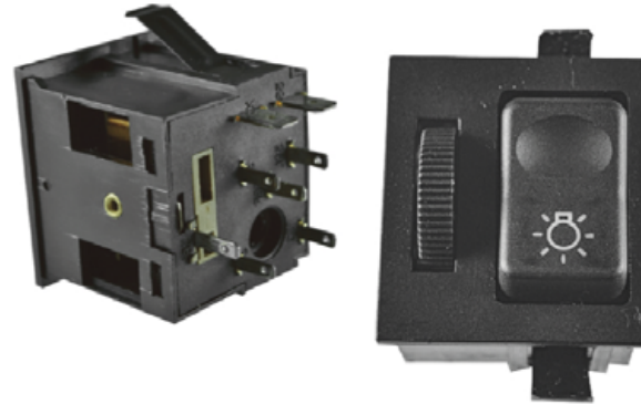
DNI2115 INTERRUPTOR - LUZ EMERGENCIA 8 TERMINALES 12V PARA: MERCEDES-BENZ
