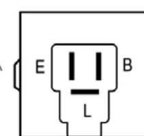
DNI1127 FLASHER 3 TERMINALES SIN SOPORTE 12V PARA: HYUNDAI, KIA, MAZDA 323-626
