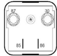
DNI8130 RELAY CON SOPORTE 12V 200A PICO (ALARMAS, BLOQUEOS, BATERIAS,LLAVE ELECTRICA) PARA: FOTON, CAIO INDUSCAR
