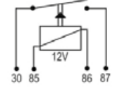
DNI8130 RELAY CON SOPORTE 12V 200A PICO (ALARMAS, BLOQUEOS, BATERIAS,LLAVE ELECTRICA) PARA: FOTON, CAIO INDUSCAR
