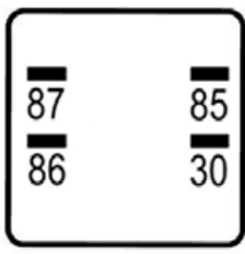
DNI8120 RELAY AUXILIAR 4 TERMINALES SIN SOPORTE TIPO AGUJA 12V 40A PARA: AVEO, SPARK, OPTRA, GM
