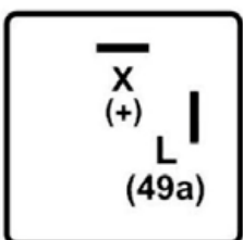
DNI1121 FLASHER 2 TERMINALES SIN SOPORTE 12V 120W
