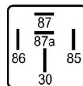
RENPREW RELAY ELECTRONICO JAPONES PARA NPR - REWARD 24V
