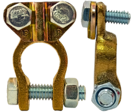
BC2L Borne Batería tipo Liviano Corriente con tornillo cabeza hexagonal Empaque X 20 UND
