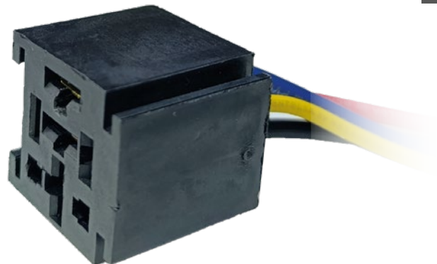
SR705B SOCKET PARA RELAY DE 80A 5 PATAS BAJITO SIN SOPORTE X5 UND
