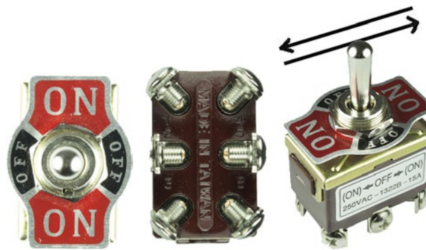
INTERRUPTOR CODILLO DE 3 CONTACTOS ON-OFF-ON EMPAQUE: 5 UND.
